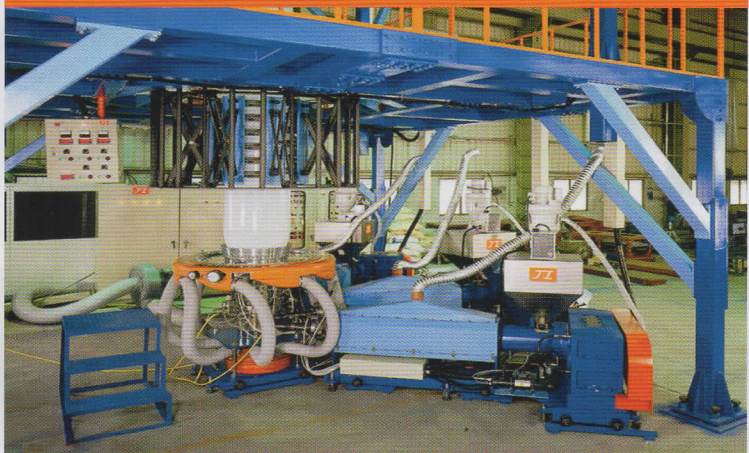
3 Layer (A-B-C) Co-extrusion 三層(A-B-C)複合吹袋
